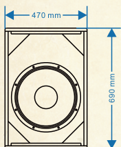
主视图
